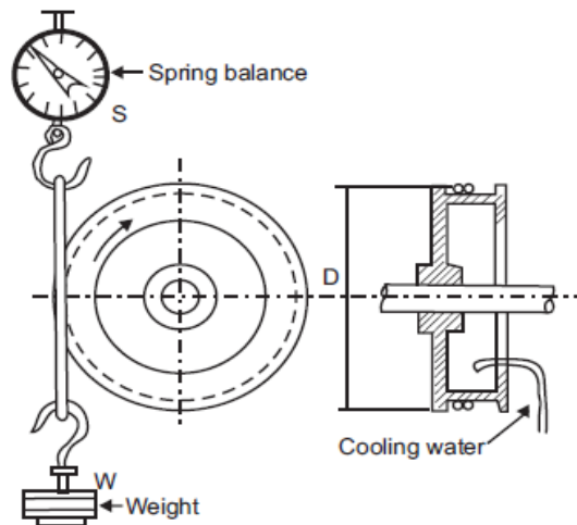
Fig. 30. Rope brake
